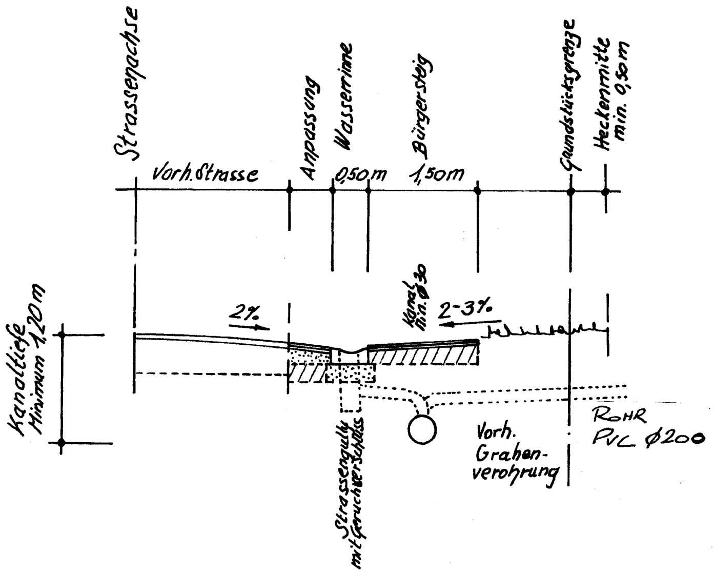
Schema Einrichtung Bürgersteig
